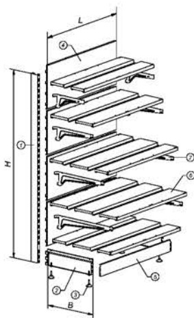
Основные элементы стеллажа «Эконом»
