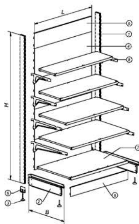
Основные элементы стеллажа «Купец»
