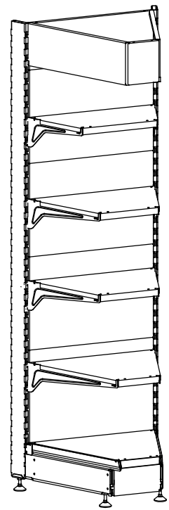
СТ4-УВ(45) Угловой внутренний 45°
